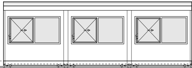
__linker zijgevel__
