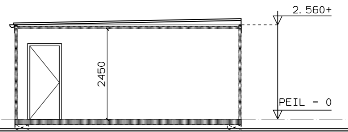
__doorsnede__
