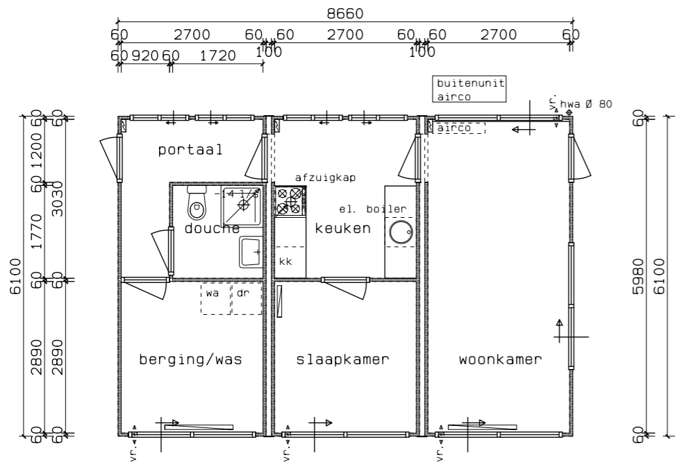
__plattegrond__
