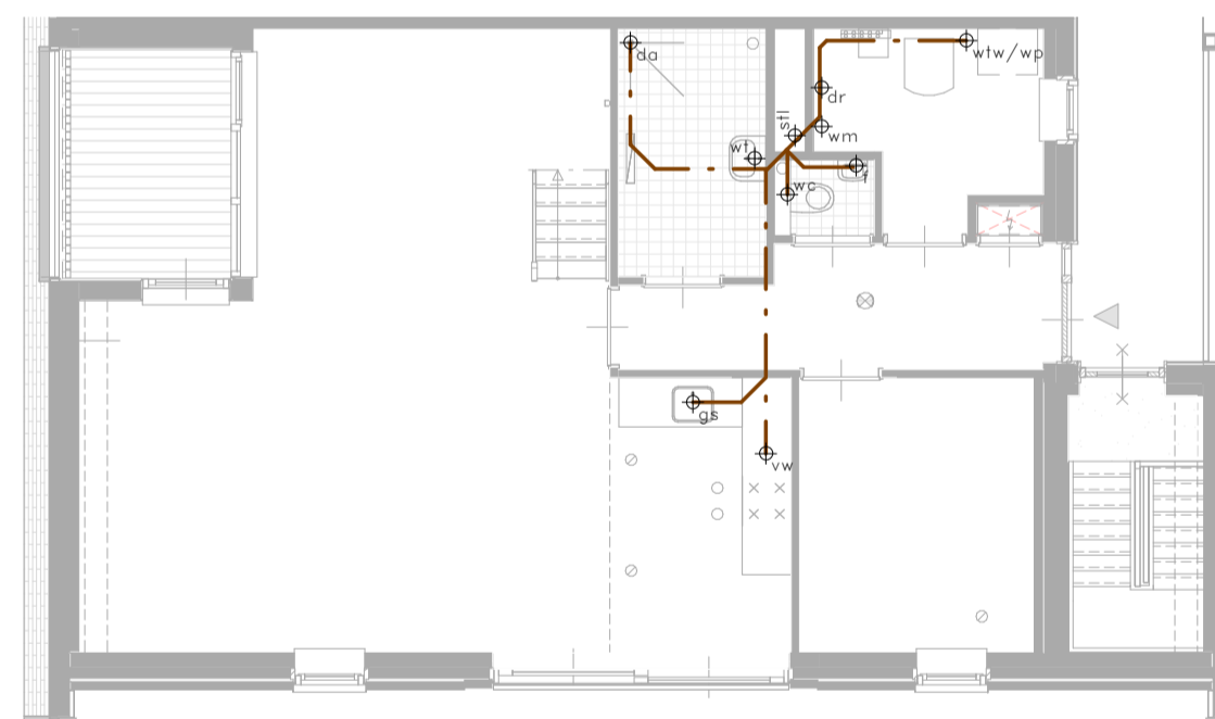
RIOLERING - TYPE B6 4e verdieping
