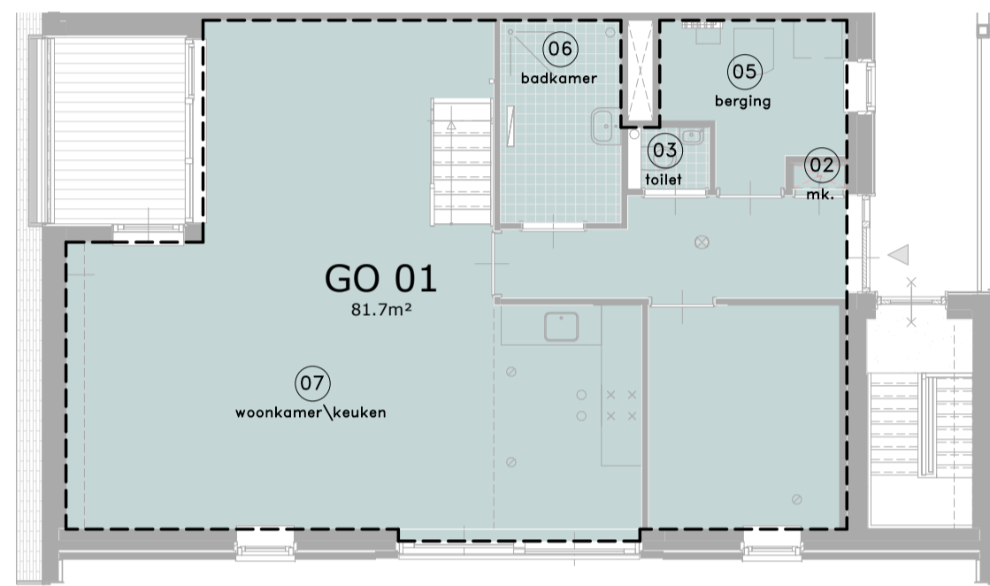
GEbruIKSOPPERVLAKTE (GO) - TYPE B6 4e verdieping
