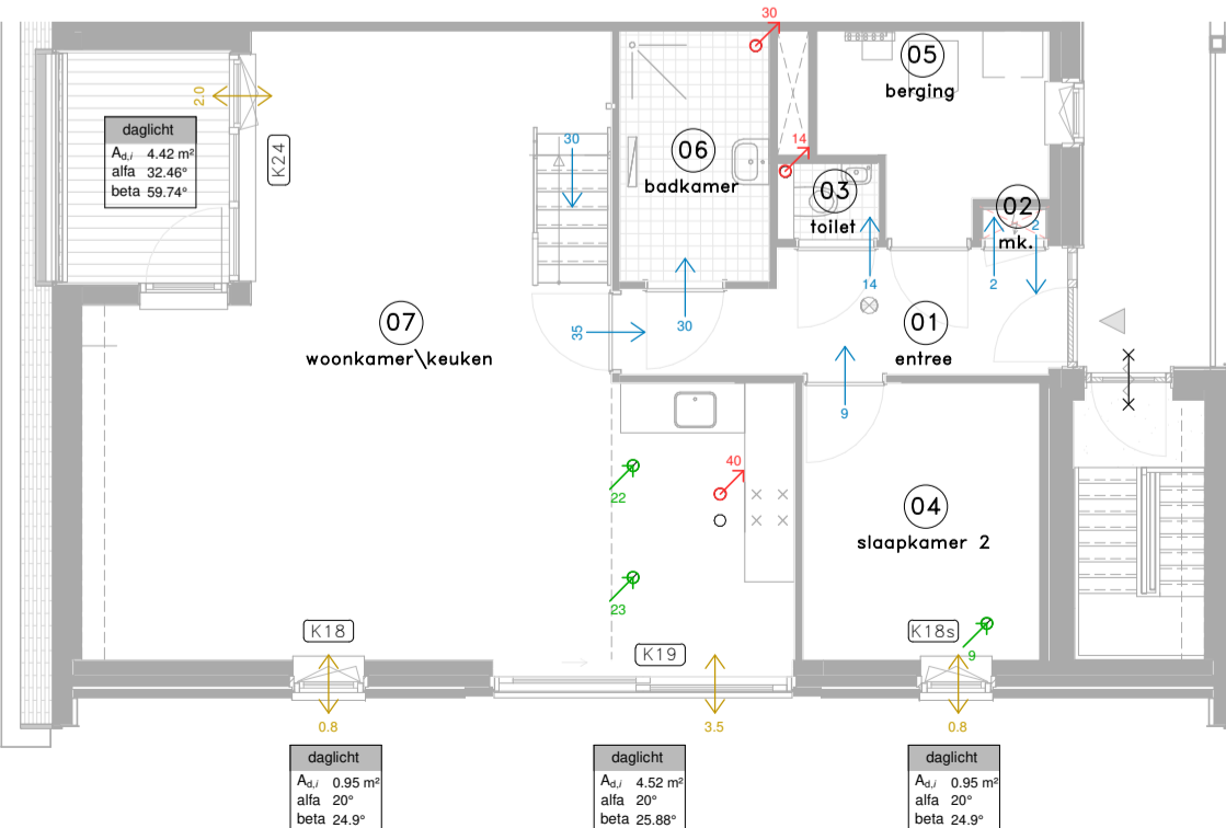
DAGLICHT + VENTILATIE - TYPE B6 4e verdieping
