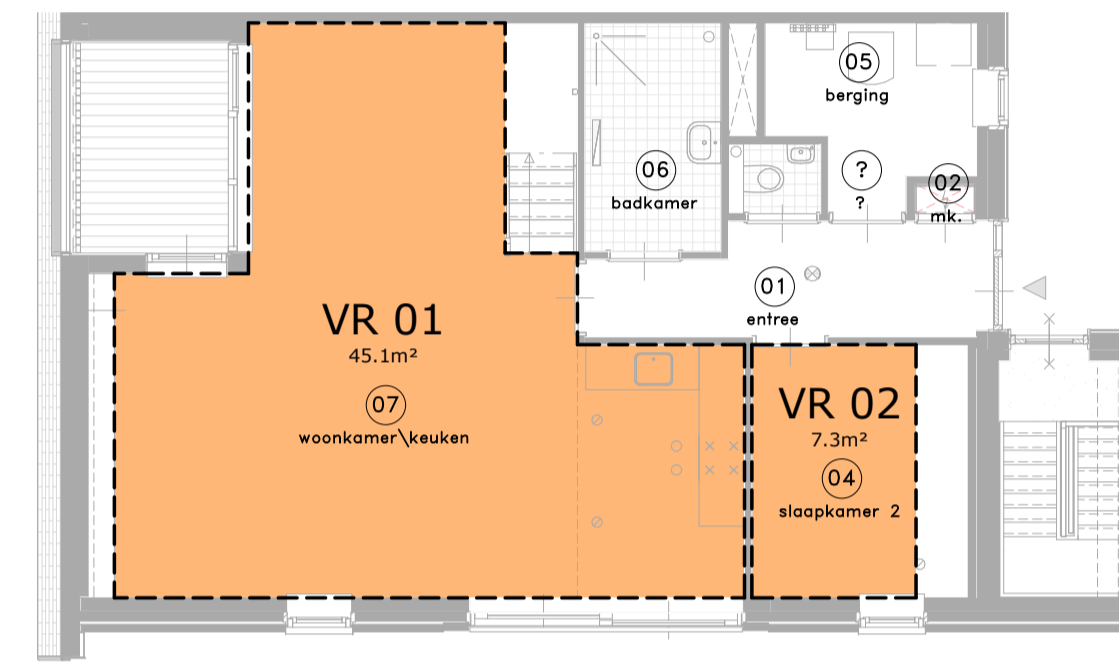
VERBLIJFSRUIMTE (VR) - TYPE B6 4e verdieping
