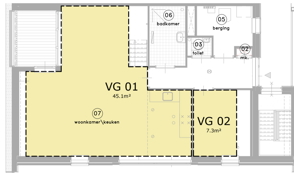
VERBLIJFSGEBIED (VG) - TYPE B6 4e verdieping
