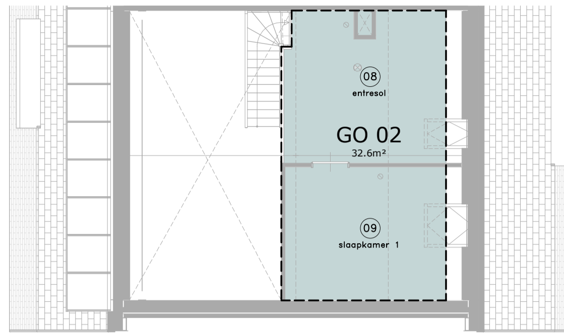
GEbruIKSOPPERVLAKTE (GO) - TYPE B6 5e verdieping
