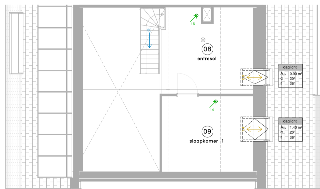
DAGLICHT + VENTILATIE - TYPE B6 5e verdieping
