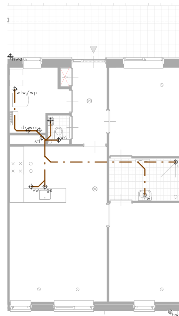
RIOLERING - TYPE A1 1e verdieping
