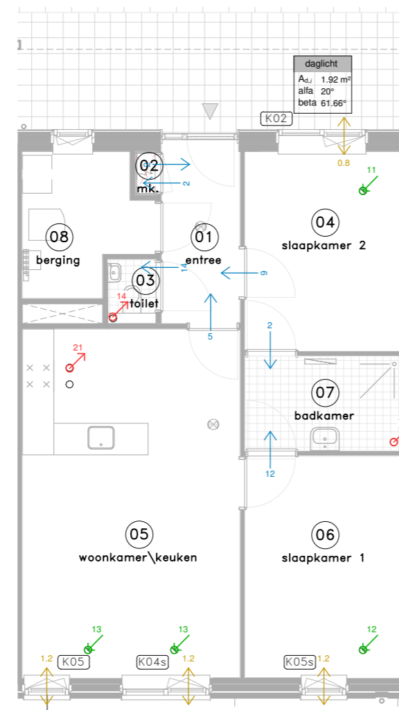
DAGLICHT + VENTILATIE - TYPE A1 1e verdieping
