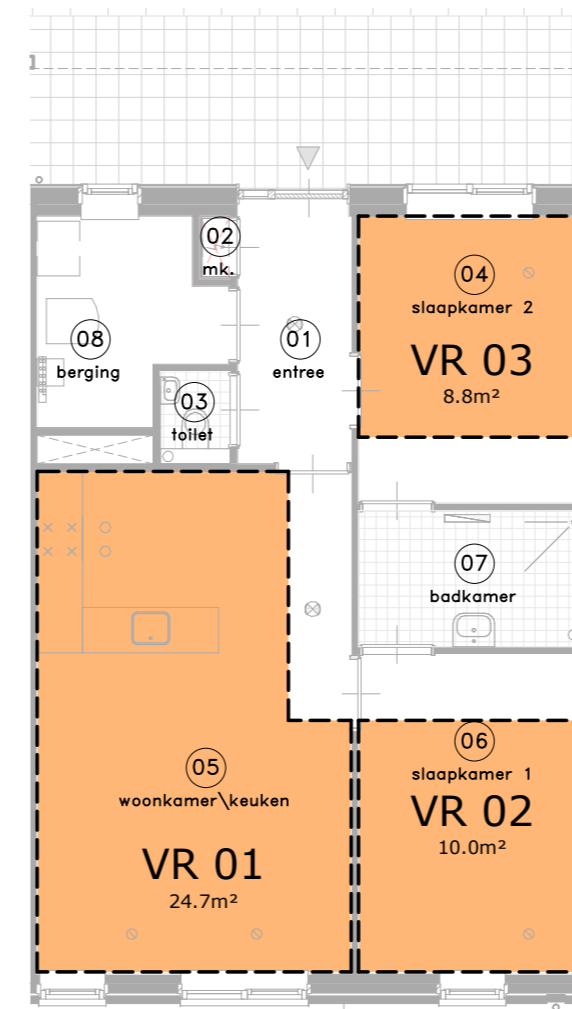
VERBLIJFSRUIMTE (VR) - TYPE A1 1e verdieping
