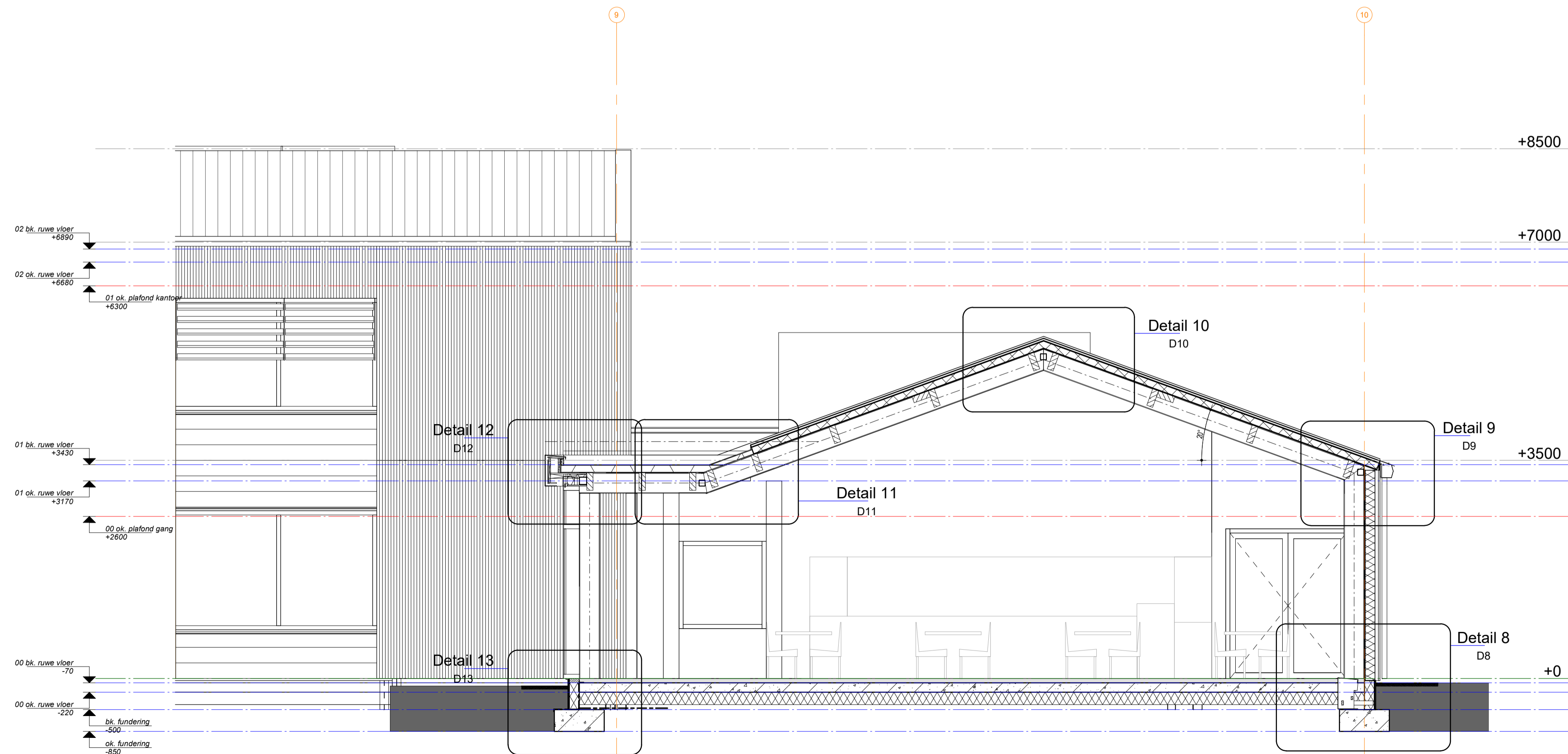
Doorsnede B1 1 : 50
